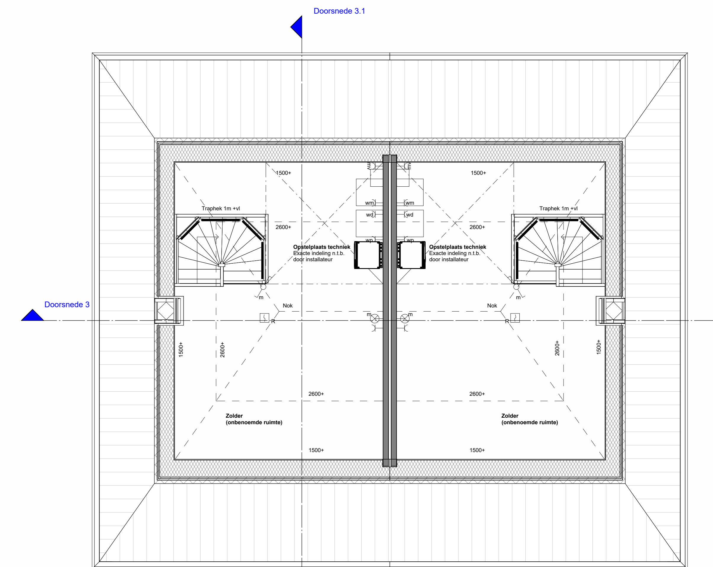
2e verdieping Schaal: 1 : 50
