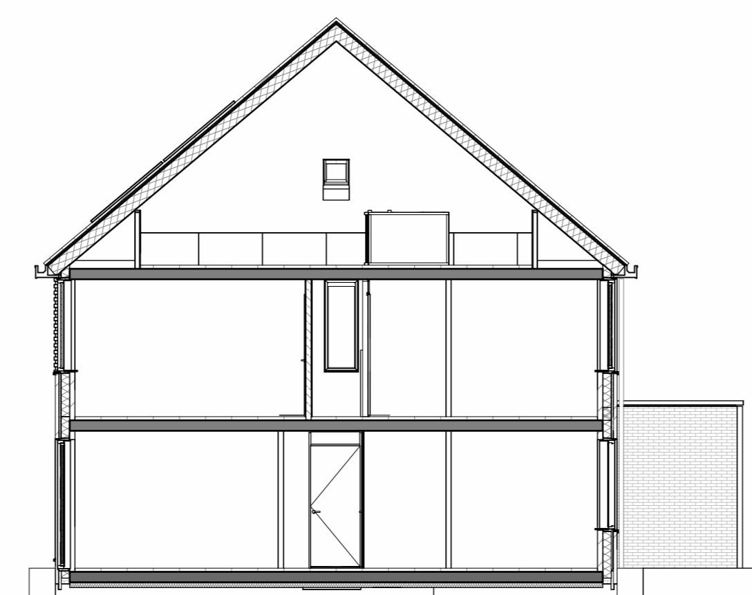
Doorsnede 3.1 Schaal: 1 : 100
