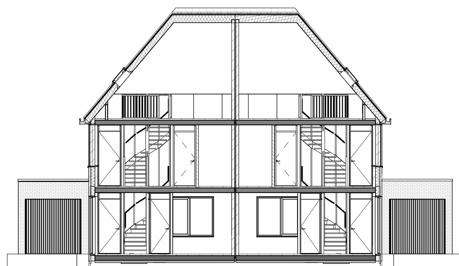
Doorsnede 3 Schaal: 1 : 100
